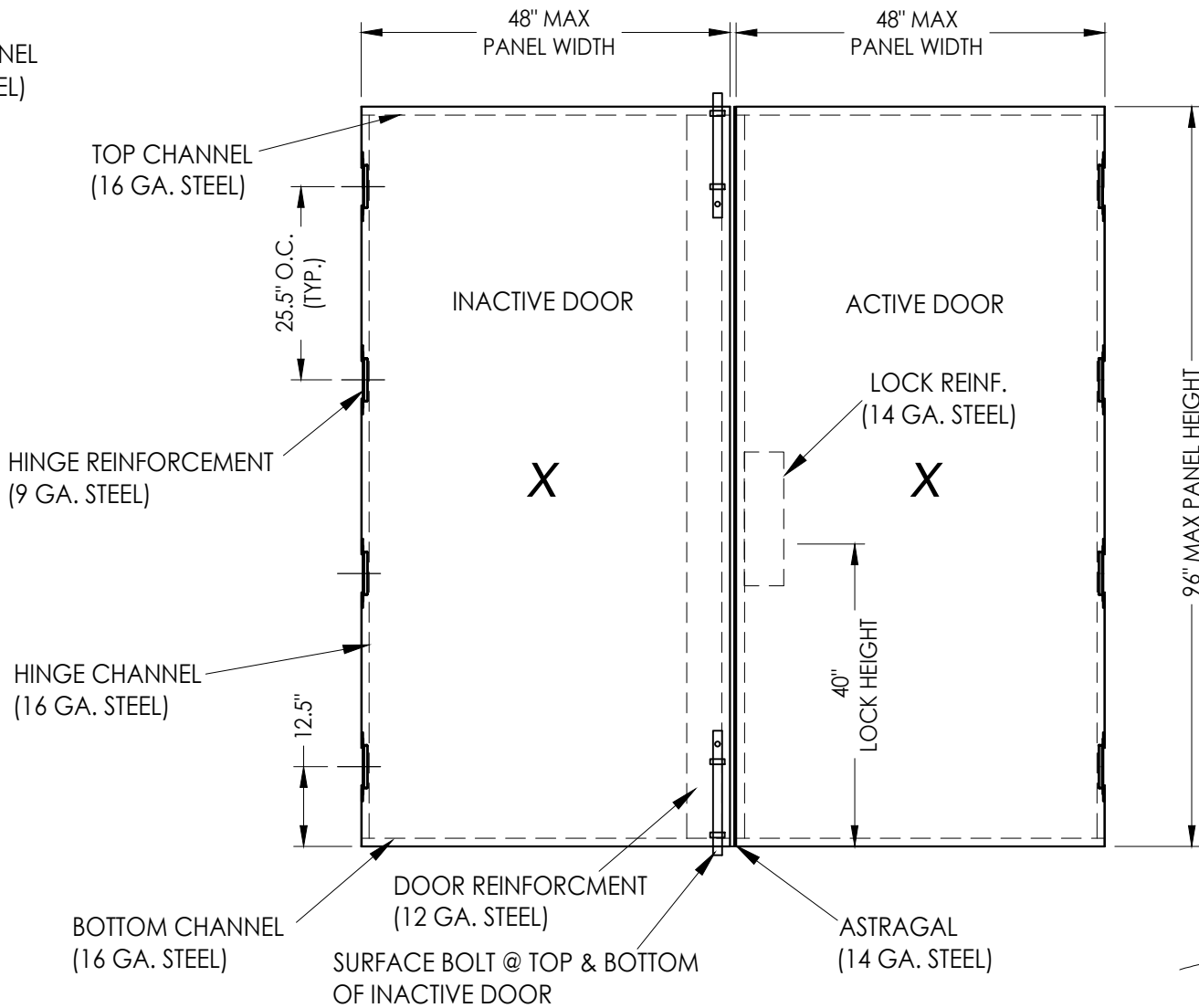
16 GAUGE STEEL DOOR PANEL (SINGLE OR DOUBLE) STEEL DOOR SKIN: MIN. 0.054" THK.
