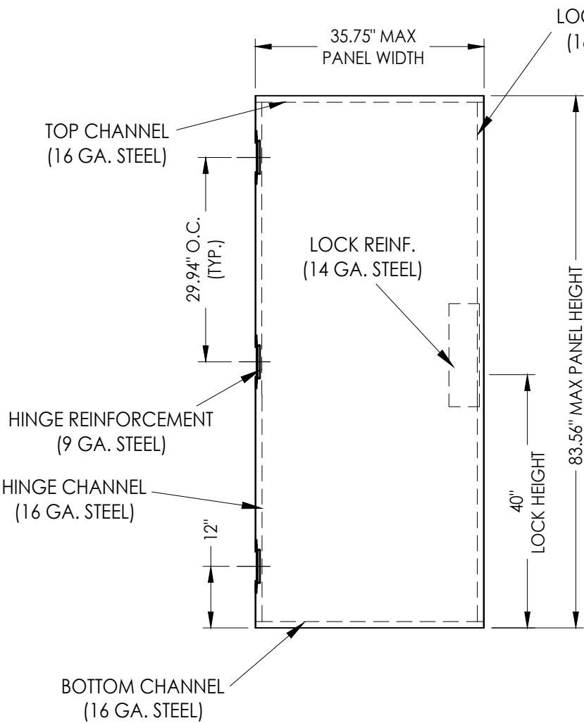
18 GAUGE STEEL DOOR PANEL (SINGLE) STEEL DOOR SKIN: 0.044" MIN. THK.
